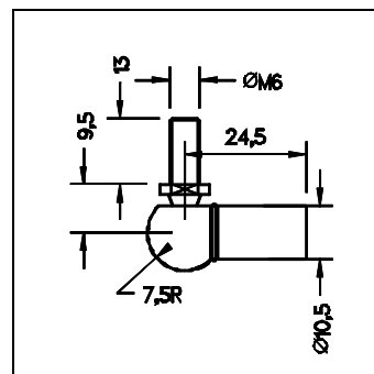
Attacco TS1 (disponibile con filetto M8)
