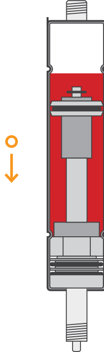
EASY KOLBENSTANGE ZEIGT NACH UNTEN PISTON ROD POINTING DOWNWARDS
